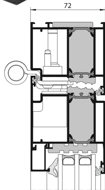
Schnittdarstellung BLECHER Alu D 72
